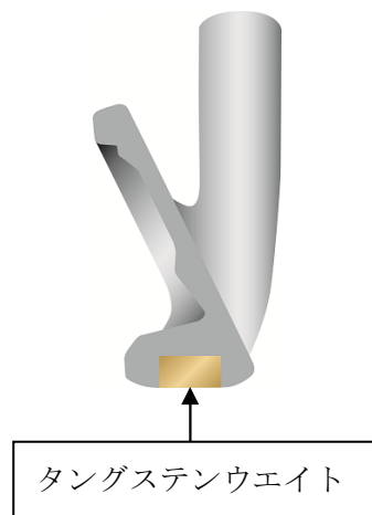
図3：タングステンを埋め込んだアイアンの断面図（イメージ）
